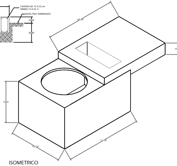
ISOMETRICO
