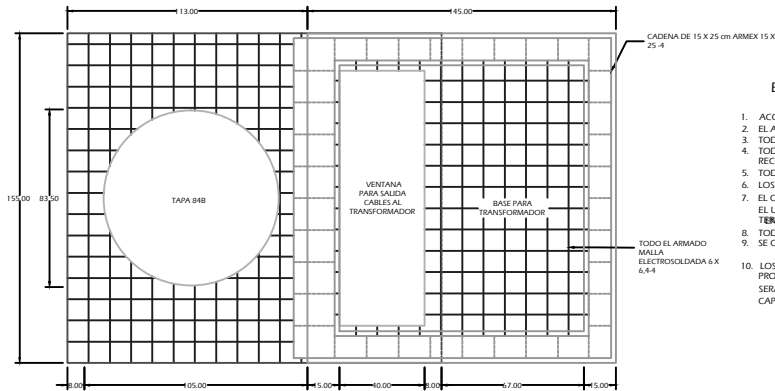
PLANTA BASE PARA TRANSFORMADOR Y REGISTRO TIPO 4 EN BANQUETA
